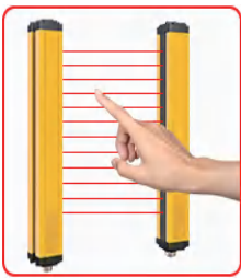
手指检测用 最小检测物体 Φ15mm (光轴间距10mm)
