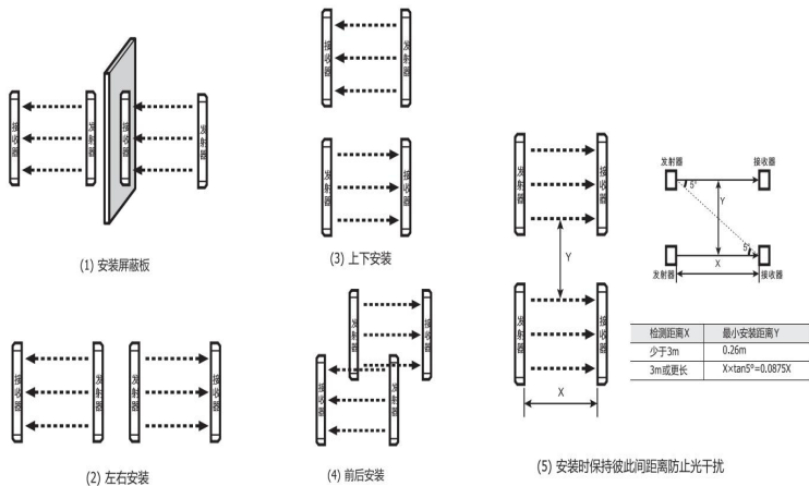
防止光栅与光栅之间相互干扰的安装位置示意图
