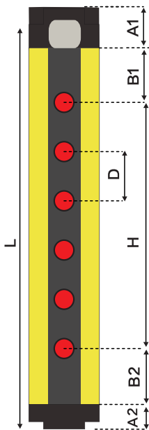
尺寸图
