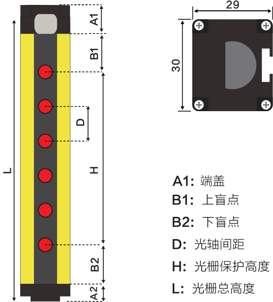
尺寸图
